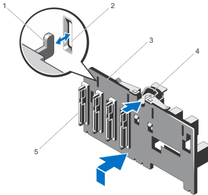
그림 57 . 2.5인치 (x4) Dell PowerEdge Express Flash(PCIe SSD) 후면판의 분리 및 설치
