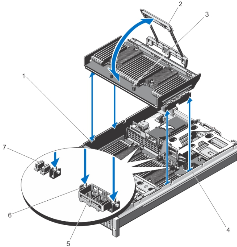
그림 12. 프로세서 확장 모듈 분리 및 설치
