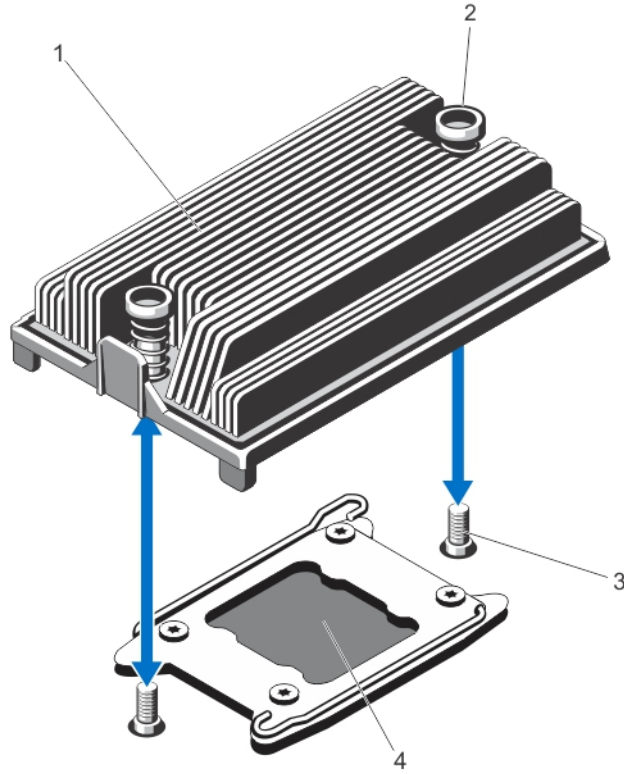
그림 44. 프로세서 방열판 분리 및 설치
