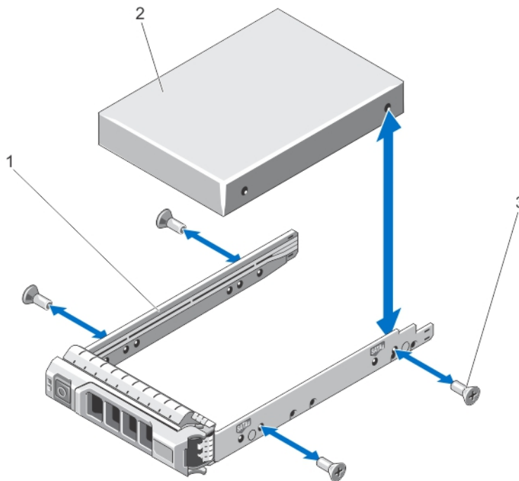
그림 20. 하드 드라이브 캐리어에서 하드 드라이브 분리 및 설치
