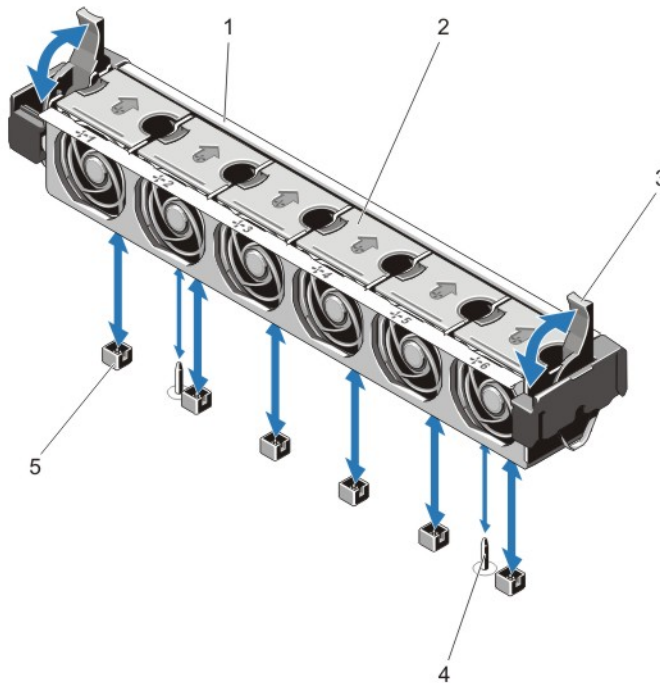
그림 23. 냉각 팬 조립품 분리 및 설치
