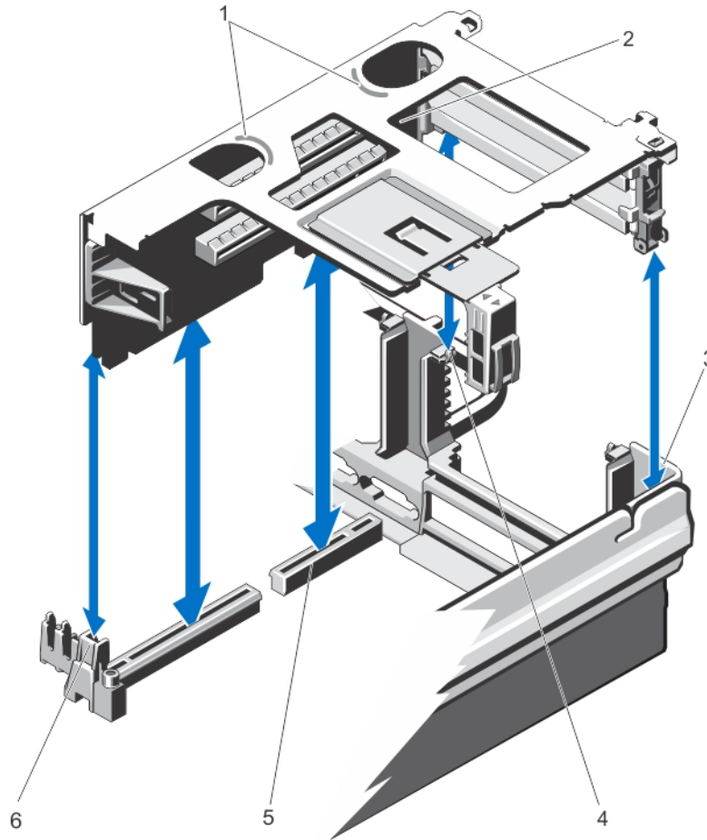
그림 30. 확장 카드 라이저 1 분리 및 설치
