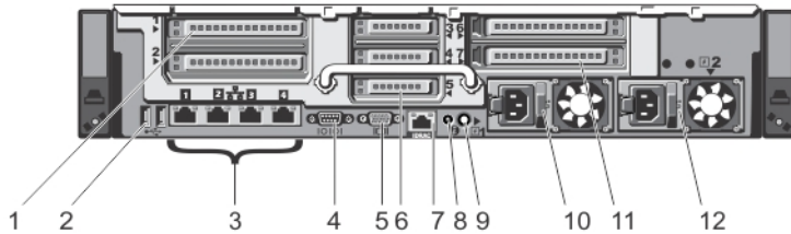
그림 4. 후면 패널 기능 및 표시등
