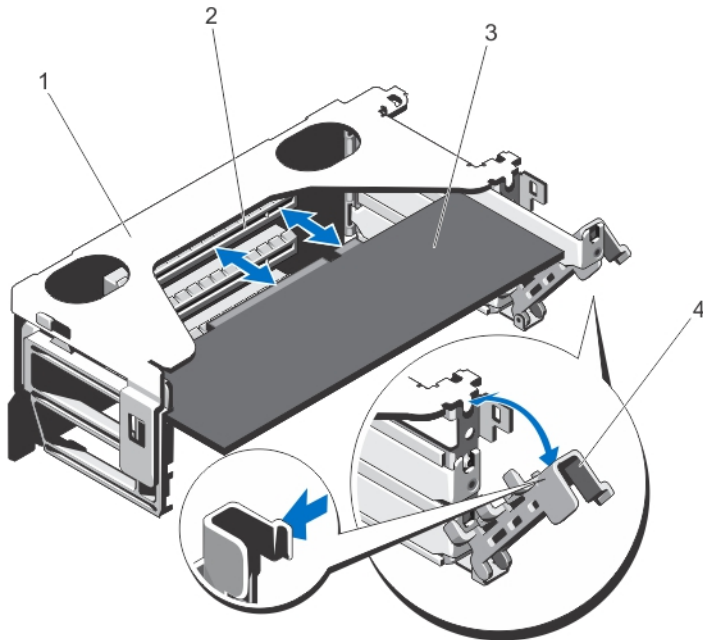
그림 27. 확장 카드 라이저 2에서 확장 카드 분리 및 설치
