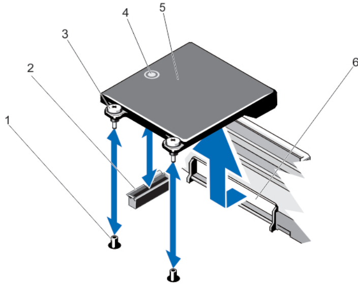
그림 43. 네트워크 도터 카드 분리 및 설치
