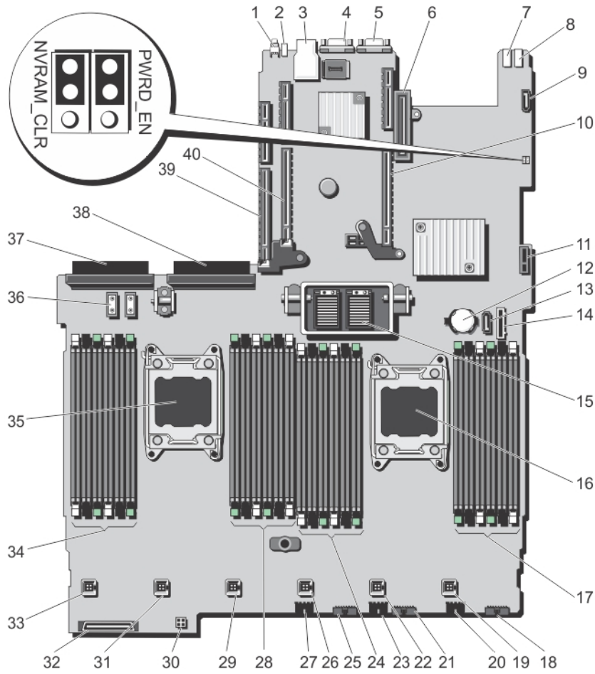
그림 66. 시스템 보드 커넥터
