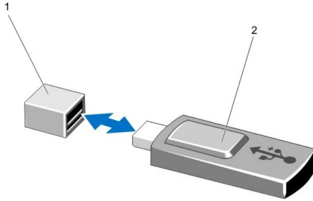
그림 24. 내부 USB 키 장착
