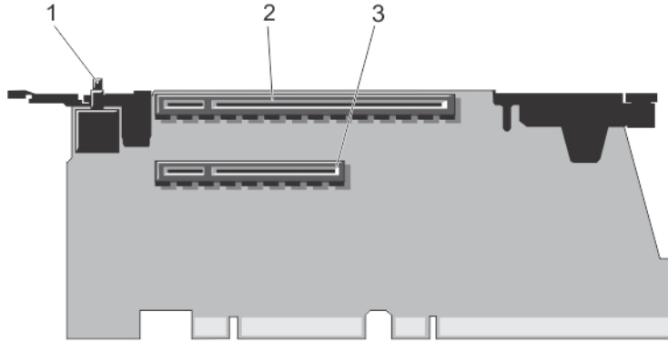
그림 35. 확장 카드 라이저 3의 커넥터
