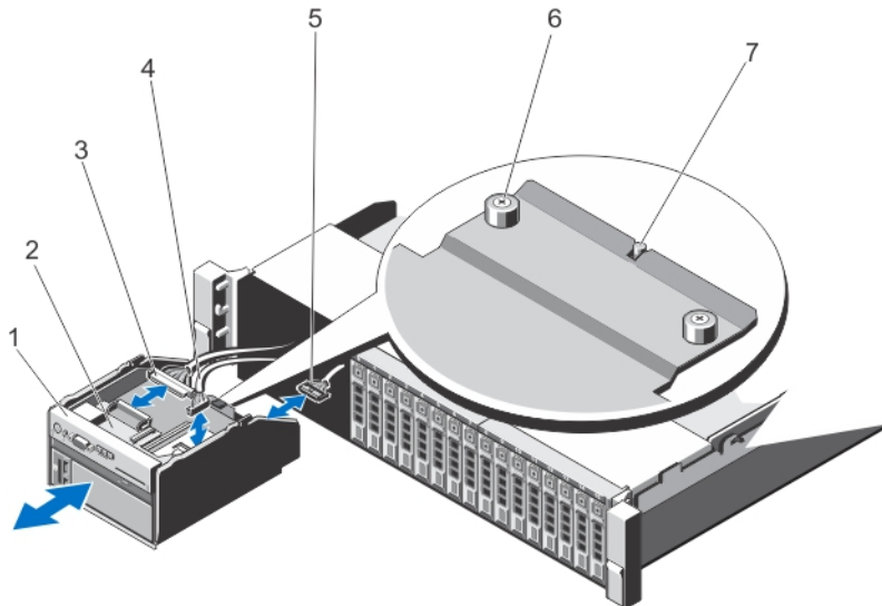
그림 63. 제어판 조립품 분리 및 설치
