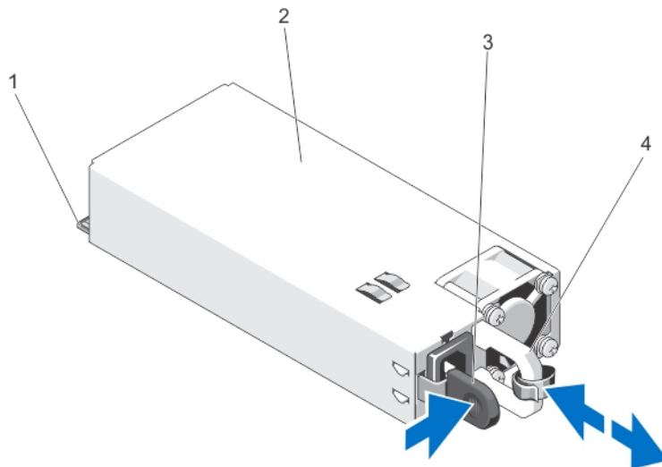
그림 47. AC 전원 공급 장치 분리 및 설치
