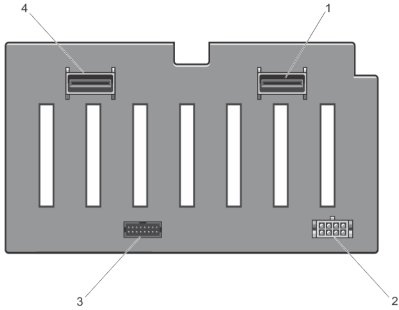
그림 54. 커넥터 다이어그램 - 2.5인치 (x8) 하드 드라이브 후면판
