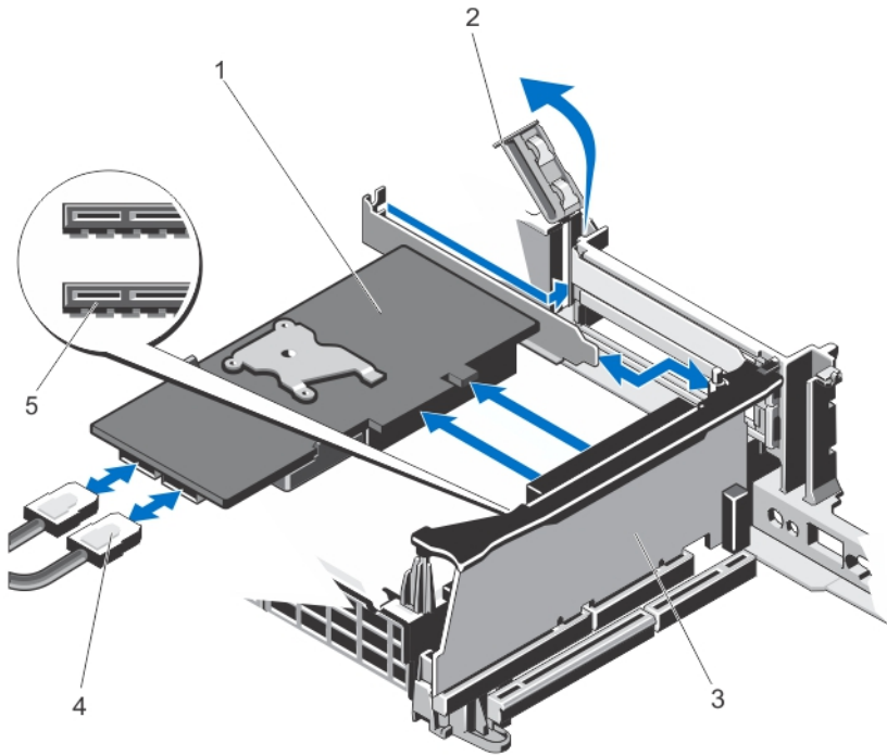
그림 39. 내장형 저장소 컨트롤러 카드 분리 및 설치
