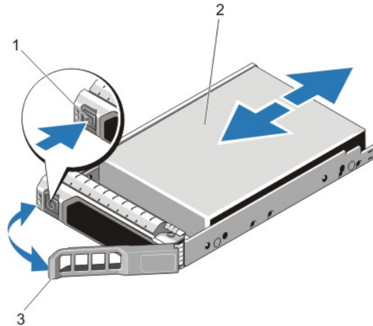
그림 19. 핫 스왑 하드 드라이브 분리 및 설치
