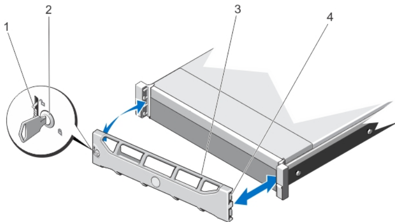
그림 8. 전면 베젤 분리 및 설치
