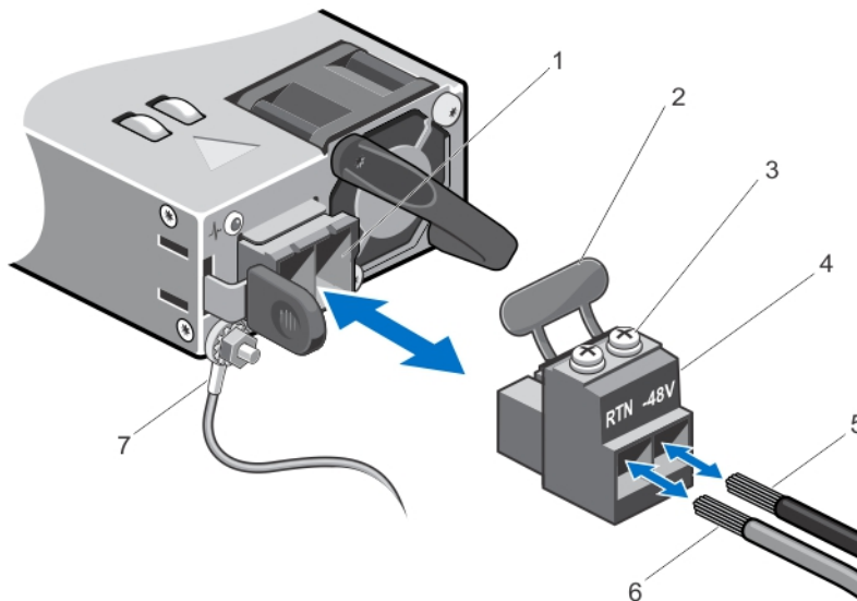
그림 49. DC 입력 전선 조립
