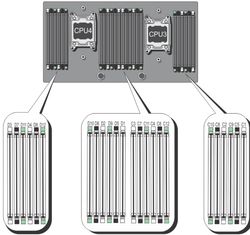
그림 16. PEM의 메모리 소켓 위치
