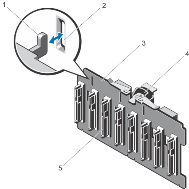
그림 53. 2.5인치 (x8) 하드 드라이브 후면판 분리 및 설치
