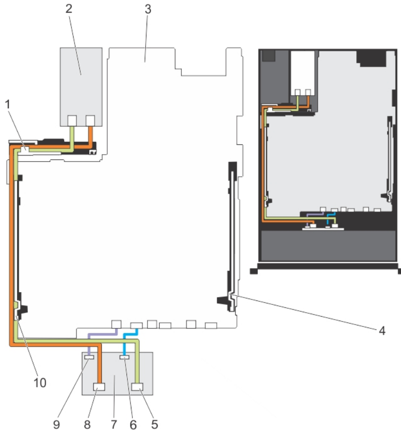
그림 55. 케이블 다이어그램 - 2.5인치 (x8) 하드 드라이브 후면판
