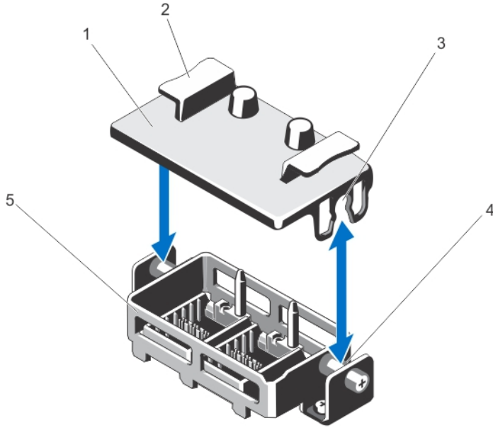
그림 13. 프로세서 확장 모듈 필러 브래킷 분리 및 설치
