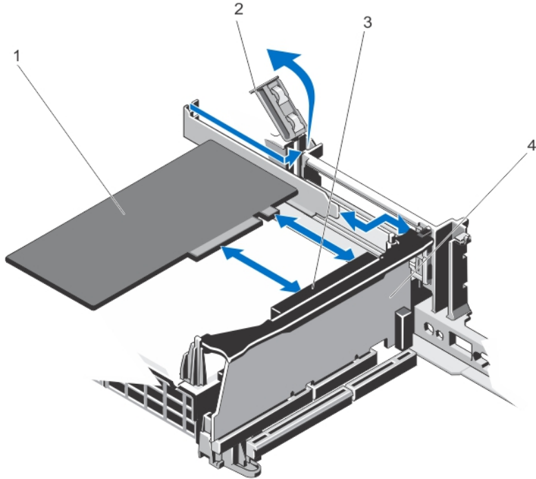
그림 28. 확장 카드 라이저 3에서 절반 높이 확장 카드 분리 및 설치
