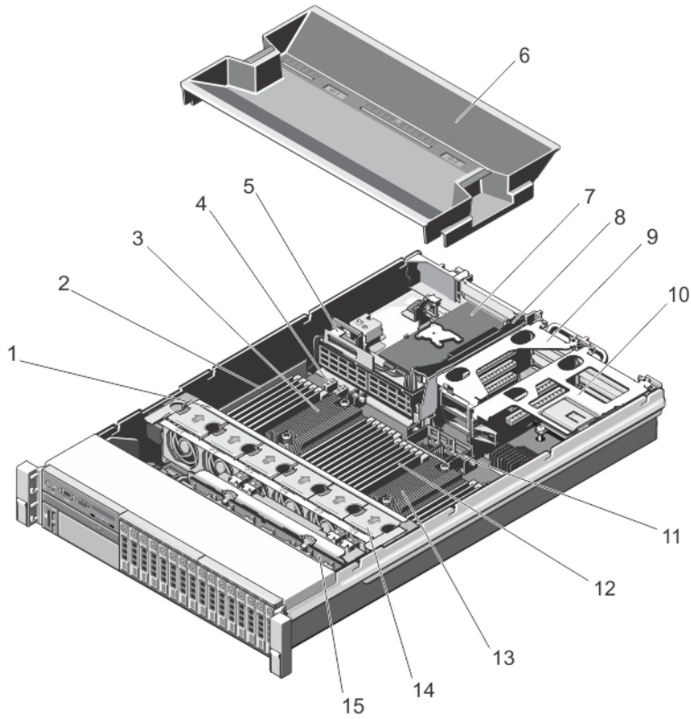
그림 10.2개 프로세서 시스템 내부
