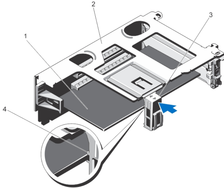
그림 26. 확장 카드 라이저 1의 확장 카드 홀더 닫기
