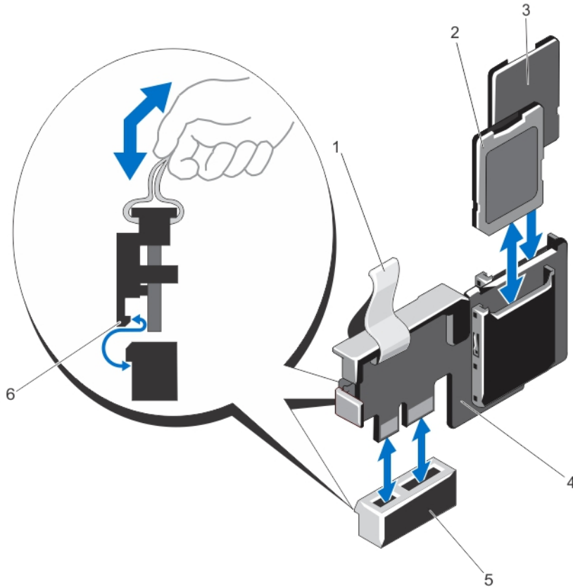
그림 37. 내부 이중 SD 모듈 분리 및 설치
