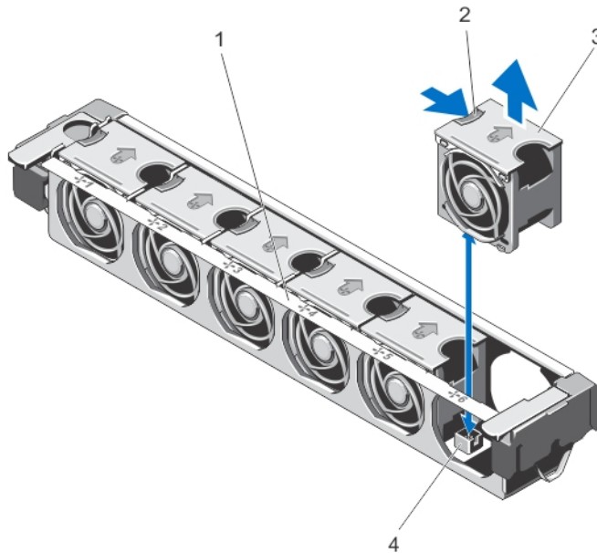
그림 22. 냉각 팬 분리 및 설치
