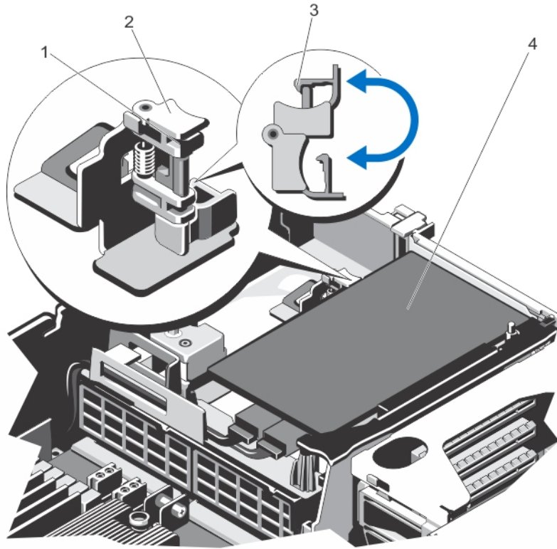
그림 29. 확장 카드 라이저 3에서 전체 높이 확장 카드 분리 및 설치
