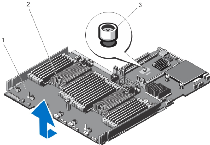
그림 65. 시스템 보드 분리 및 설치
