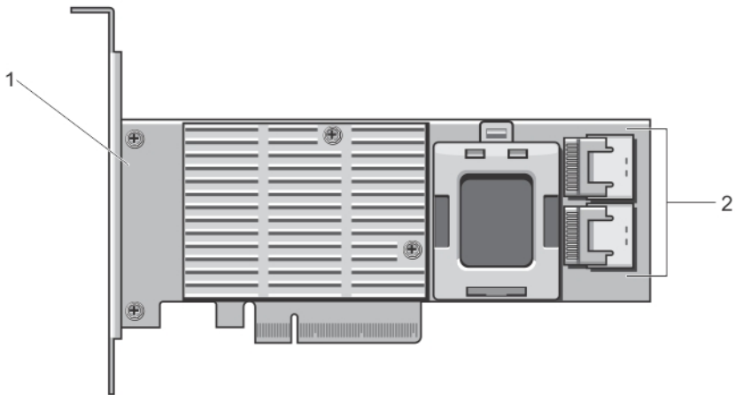
그림 40. 내장형 저장소 컨트롤러 카드의 커넥터
