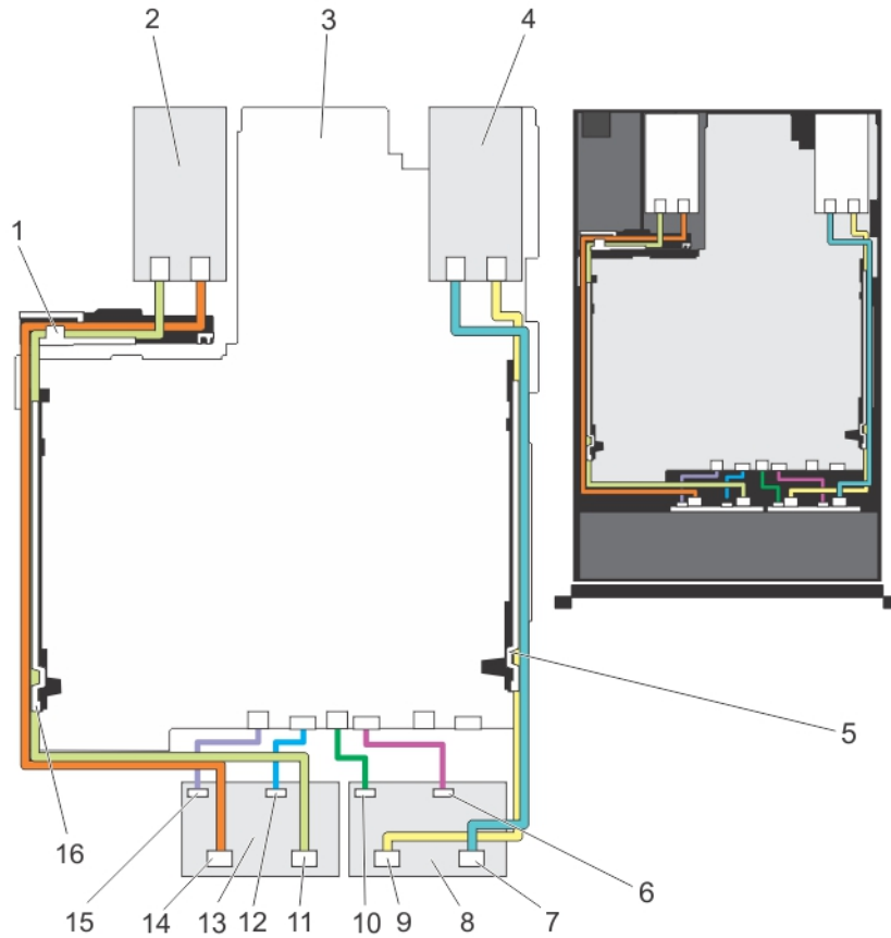
그림 56. 케이블 다이어그램 - 이중 2.5인치 (x8) 하드 드라이브 후면판
