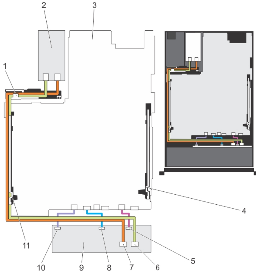
그림 62. 케이블 다이어그램 - 2.5인치 (x16) 하드 드라이브 후면판
