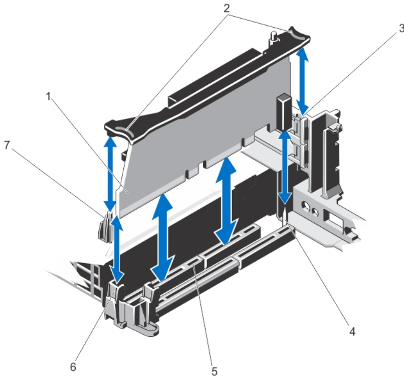
그림 34. 확장 카드 라이저 3 분리 및 설치
