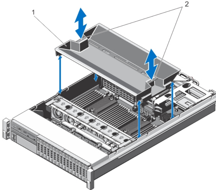
그림 14. 냉각 덮개 분리 및 설치
