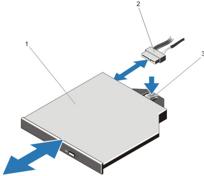
그림 21. 광학 드라이브 분리 및 설치
