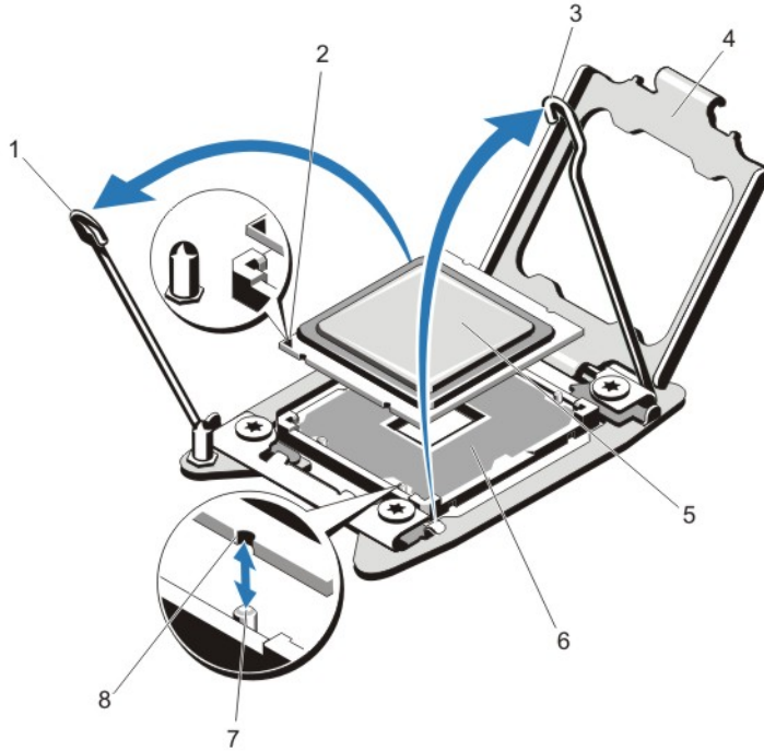
그림 46. 프로세서 분리 및 설치
