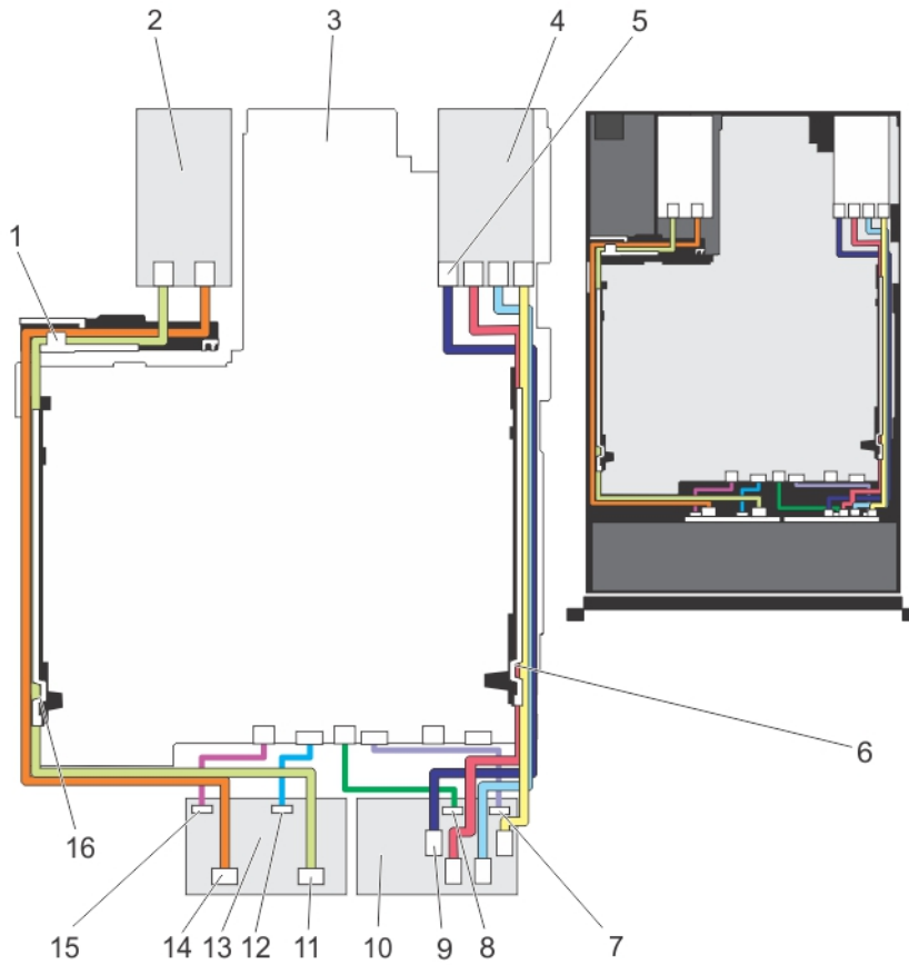
그림 59. 케이블 다이어그램 - 2.5인치 (x8) SAS/SATA 하드 드라이브 및 (x4) PCIe SSD 후면판
