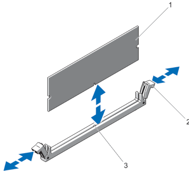
그림 17. 메모리 모듈 또는 메모리 모듈 보호물 설치 및 분리
