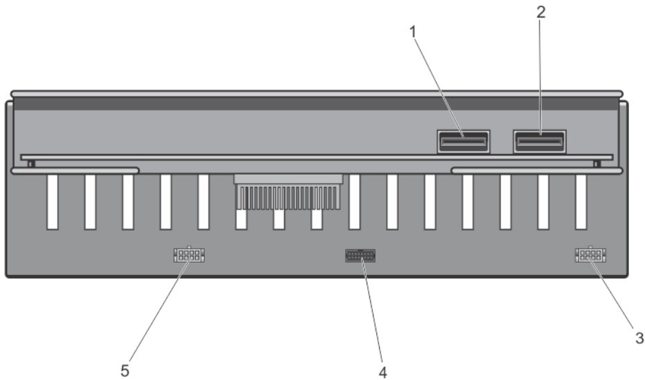
그림 61. 커넥터 다이어그램 - 2.5인치 (x16) 하드 드라이브 후면판
