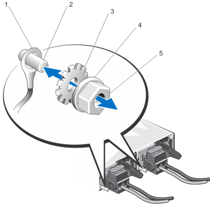
그림 48. 안전 접지선 조립 및 연결
