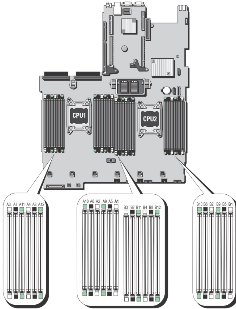
그림 15. 시스템 보드의 메모리 소켓 위치
