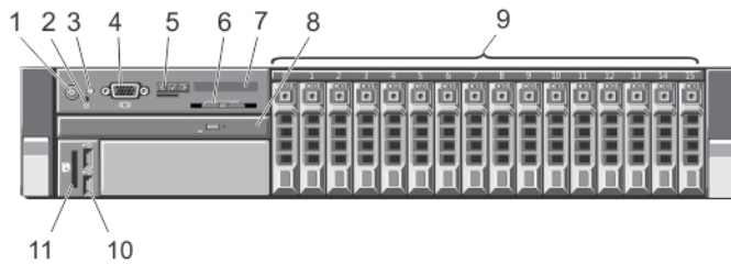
그림 1. 전면 패널 기능 및 표시등 - 16 하드 드라이브 시스템
