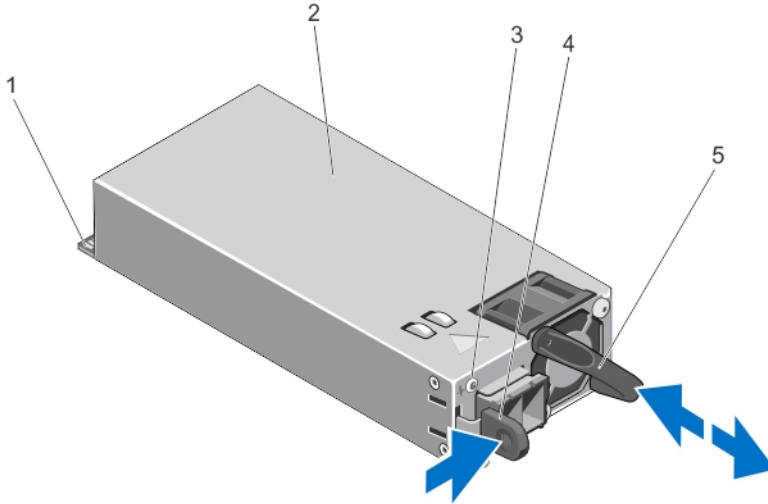
그림 50. DC 전원 공급 장치 분리 및 설치
