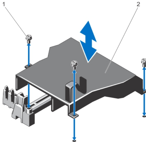
그림 42. PCH 덮개 분리 및 설치
