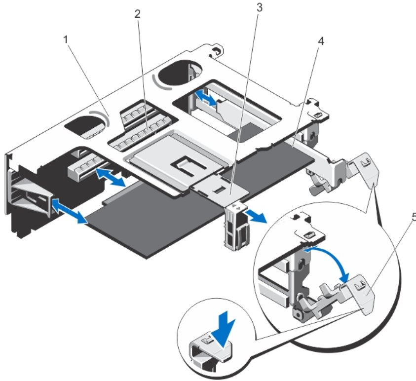
그림 25. 확장 카드 라이저 1에서 확장 카드 분리 및 설치
