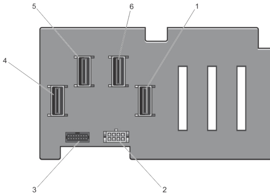
그림 58 . 커넥터 다이어그램 - 2.5인치 (x4) PCIe SSD 후면판
