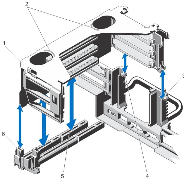
그림 32. 확장 카드 라이저 2 분리 및 설치
