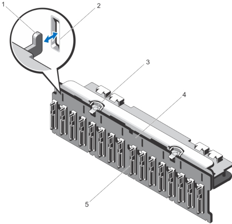
그림 60. 2.5인치 (x16) 하드 드라이브 후면판 분리 및 설치
