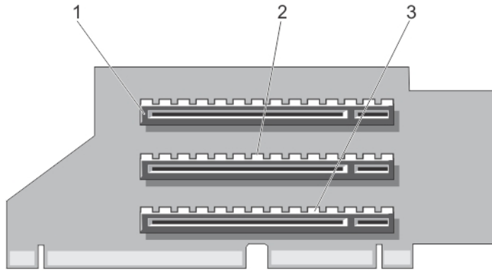
그림 33. 확장 카드 라이저 2의 커넥터
